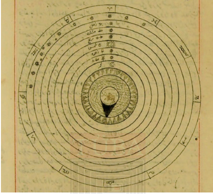
Şekil 12: Cihânnümâ'da Felekler
